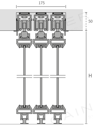
内嵌式三轨三扇吊滑门
