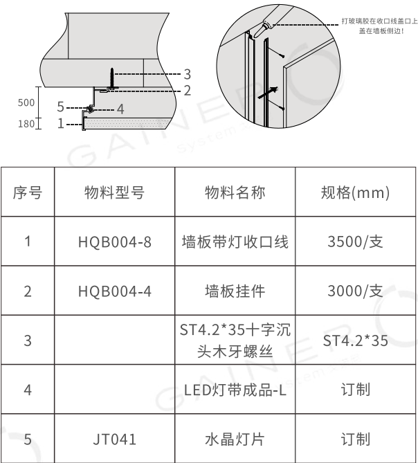
▼ 阳角收口结构设计图
