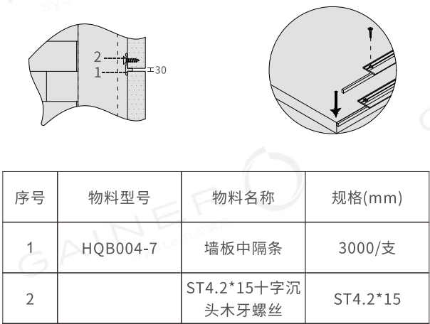
▼ 腰线分隔结构设计图
