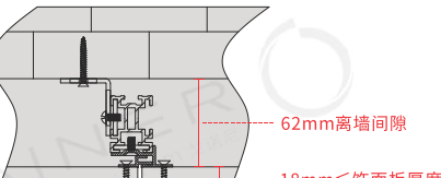
墙板离墙最大值62mm
