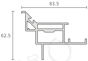
STM019-2 外平内开主套
