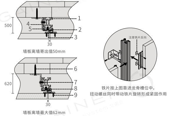
▼ 龙骨结构设计图
