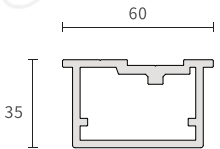
STM019-10 插销位门扇横框
