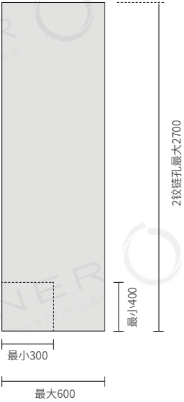
门板尺寸工艺图
