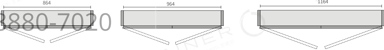
标准双门内空尺寸
