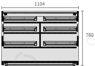
侧视图
