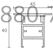
MK133-8B-2 门扇边框-拉手位
