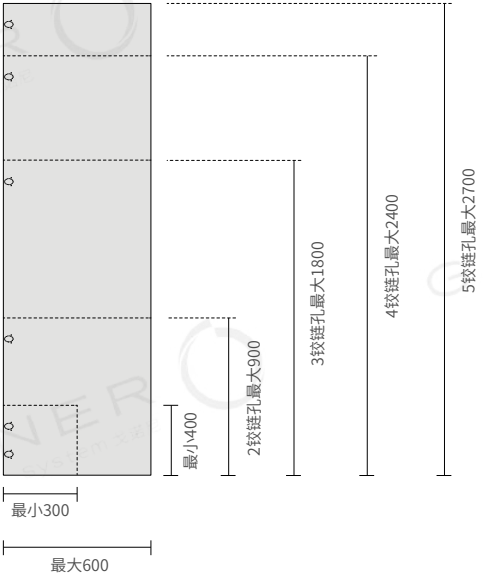
门板尺寸工艺图
