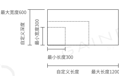
MK004尺寸范围
