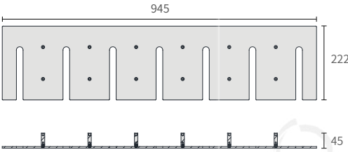
JBJ-945 标准1000柜
