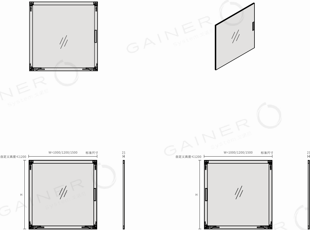
移门规格可定制 (左拉手)
