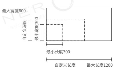
MK130尺寸范围
