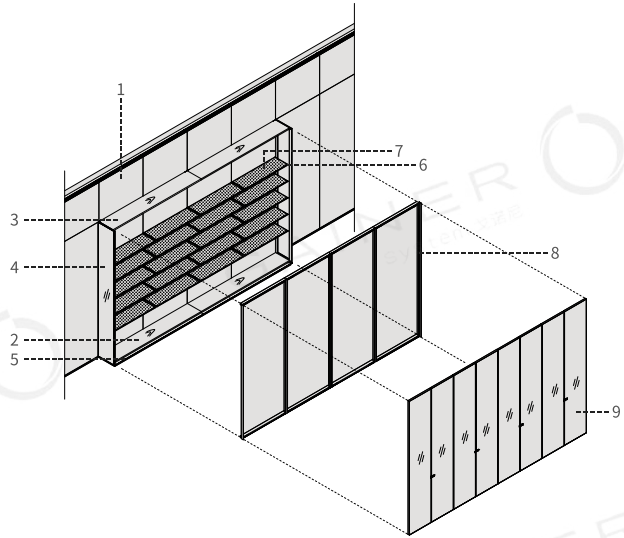
产品内部结构图
