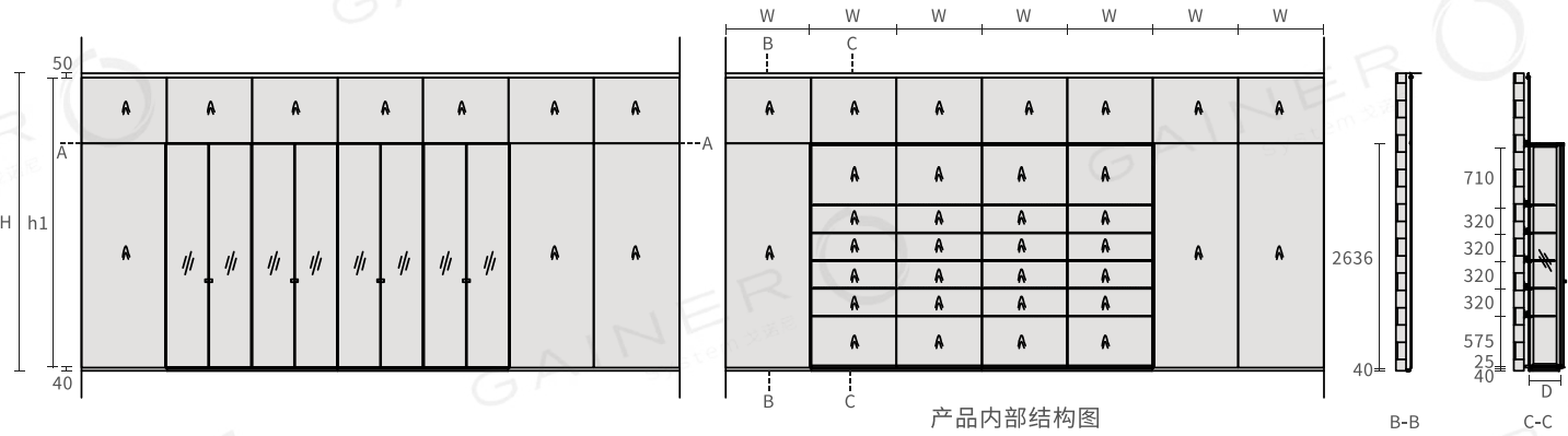
产品内部结构图
