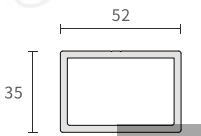
STM019-6 门扇横框
