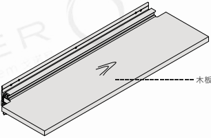
悬挑木层板 HQB005A
