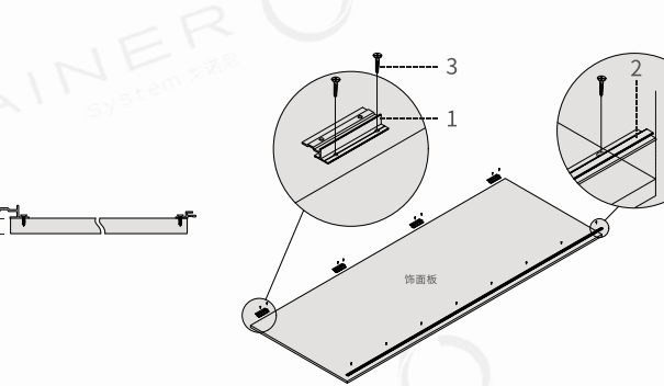
▼饰面板装配结构设计图
