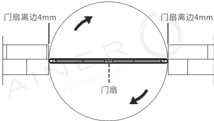
单门旋转开启
