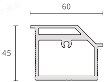
STM019-4 门扇竖框
