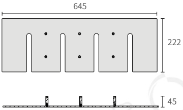
JBJ-645 标准700柜
