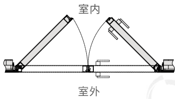
C/D 外平内开
