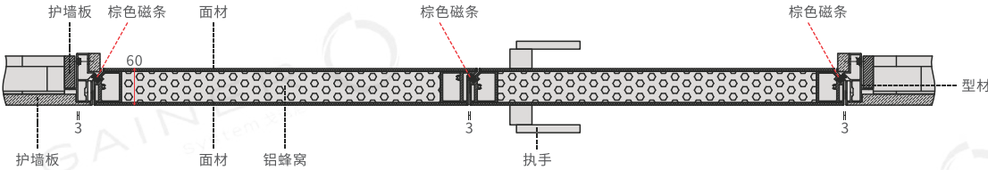
▼ A/B向门扇俯视图截面
