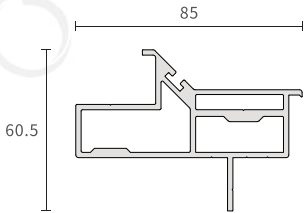
STM019-1 外平外开主套
