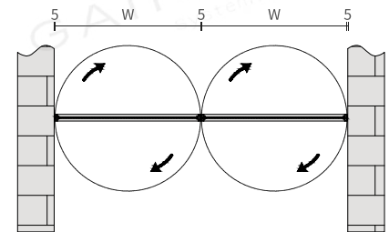
双门旋转开启
