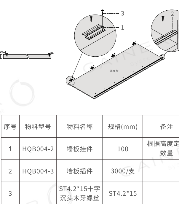
▼ 饰面板装配结构设计图
