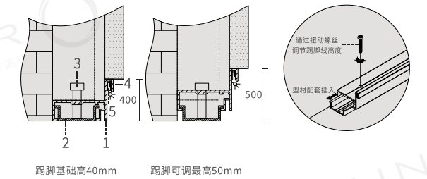
▼ 踢脚线结构设计图
