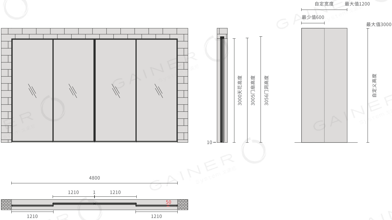
展会样品门洞尺寸(W4800*H3056)
