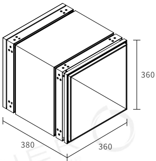
360*360 标准尺寸小模块
