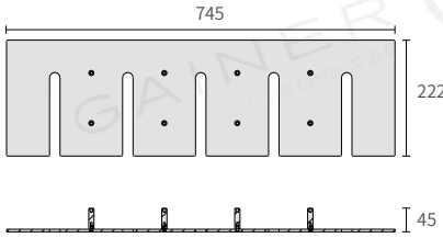
JBJ-745 标准800柜
