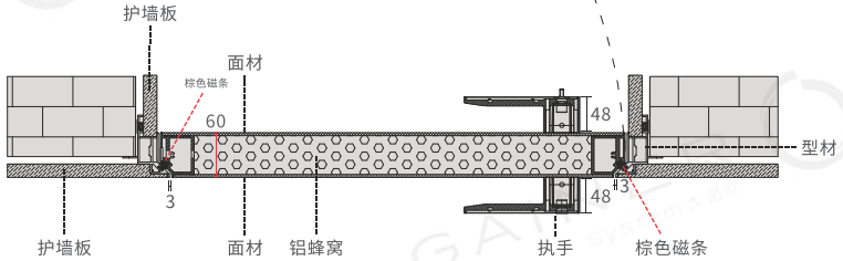
▼ D向门扇俯视图截面
