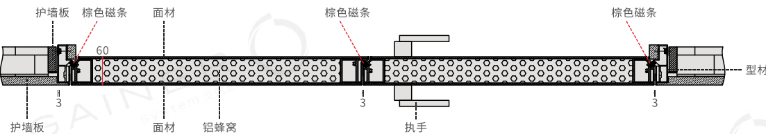
▼ A/B向门扇俯视图截面
