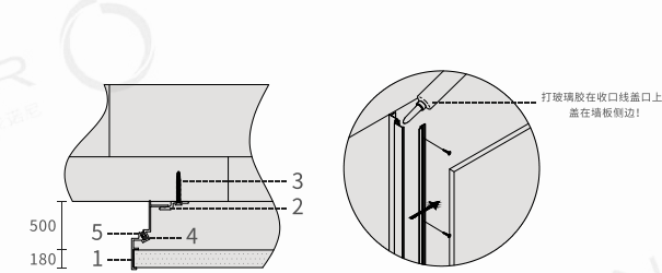
▼阳角收口结构设计图
