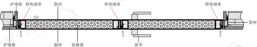
▼ C/D向门扇俯视图截面
