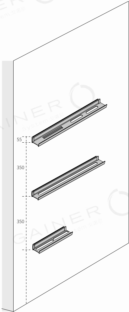
可定制安装间距, 建议使用350mm
