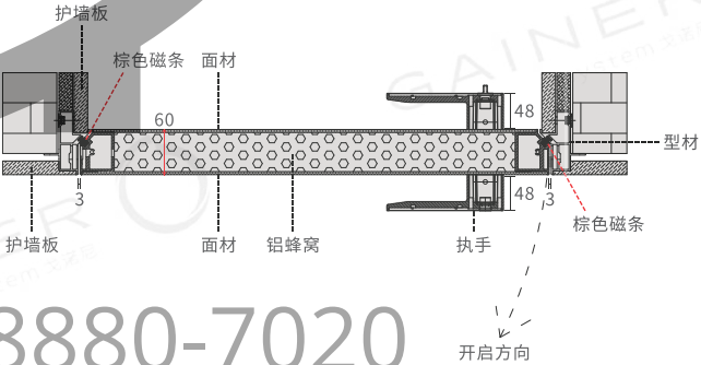
▼ C/D向门扇俯视图截面
