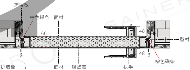
▼ B向门扇俯视图截面
