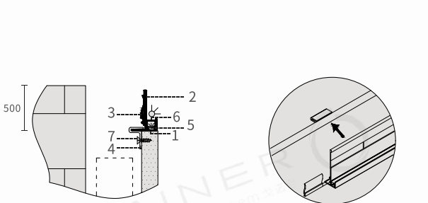
▼顶线收口结构设计图
