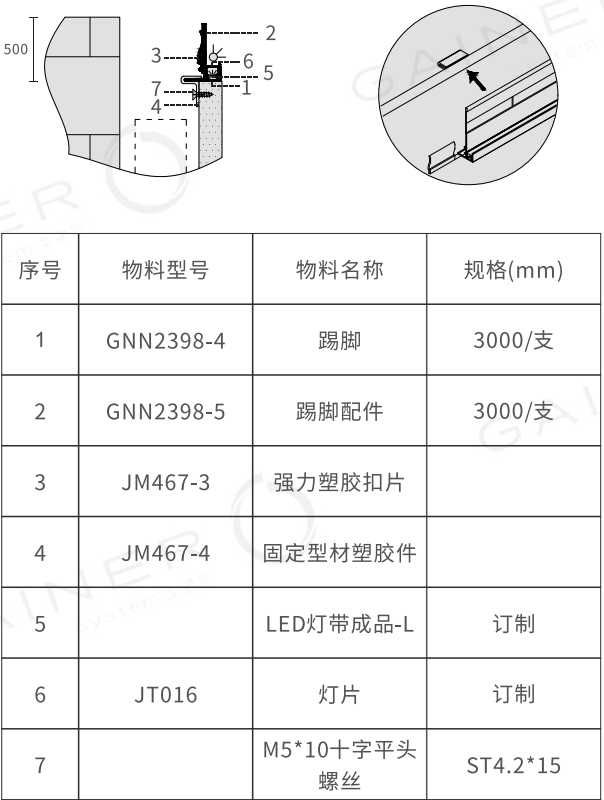
▼ 顶线收口结构设计图
