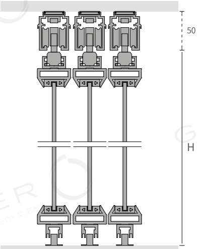
外露式三轨三扇吊滑门
