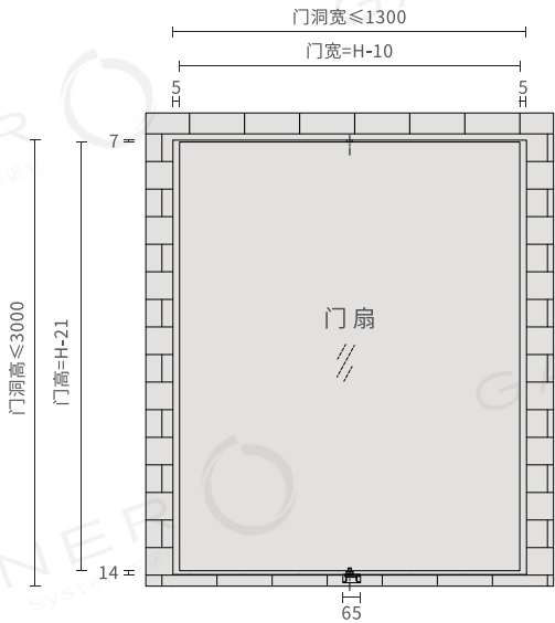
电动中轴门，带防夹手功能
