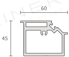
STM019-3 门扇竖框带槽
