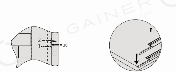
▼腰线分隔结构设计图
