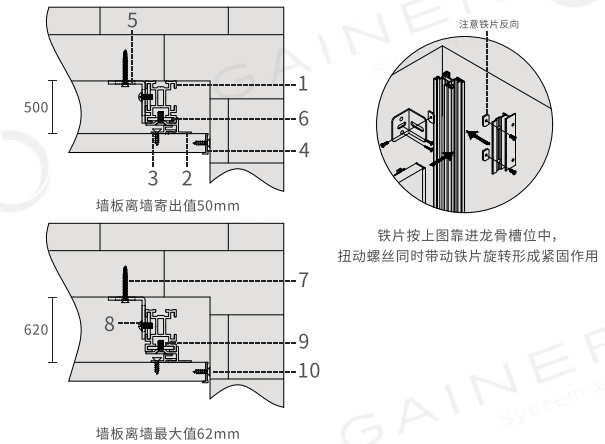
▼ 阴角收口结构设计图
